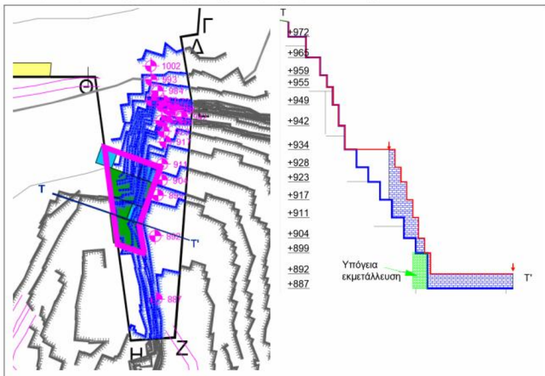
Εικόνα 4. Κατακόρυφη τομή T-T' στη θέση των υπογείων όπου φαίνονται οι διαστάσεις των υπαίθριων βαθμίδων (ύψος 12m και πλάτος 6m στη θέση της εισόδου).
