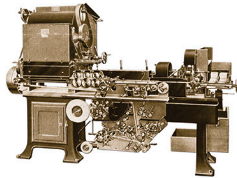
Μηχανή παραγωγής τσιγάρων. Cigarette production machine.
